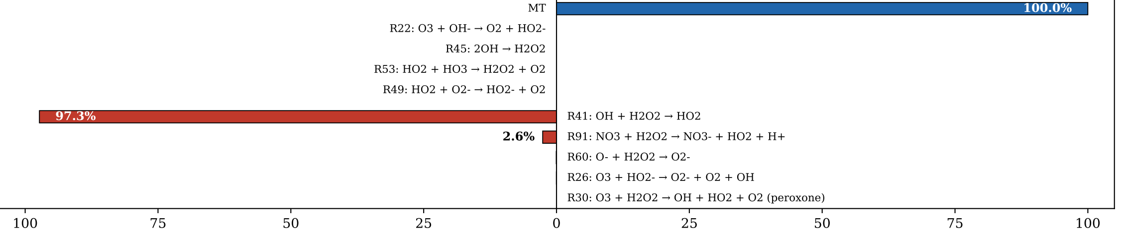
(d) H 2 O 2 (Σsrc = 3.00e-08 M/s)
